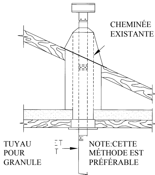
FIGURE 11 Évacuation dans une cheminée existante
