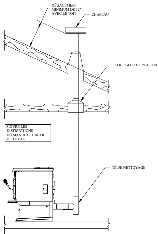
FIGURE 9 Évacuation par le toit
