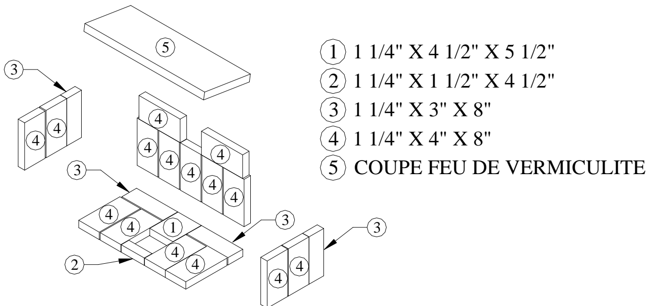
Figure 5.6.2 (B) - Disposition des briques
