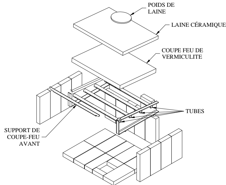
Figure 5.6.2 (A) - Installation du coupe-feu
